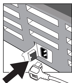
1. インレットプラグを電源差込口に接続
